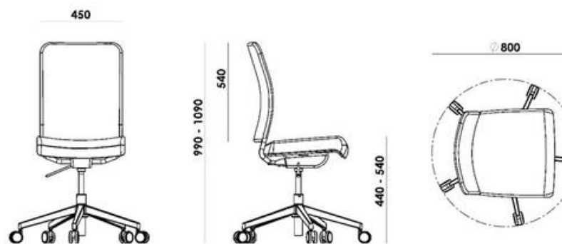
elevação frontal
