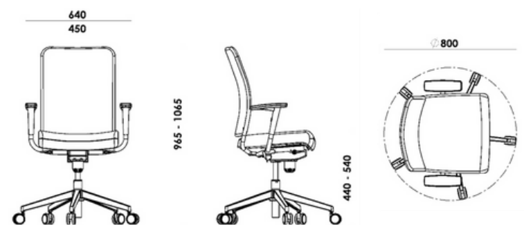
elevação frontal
